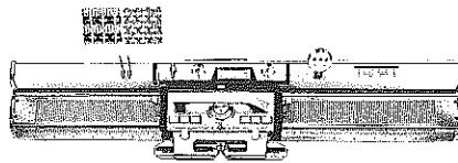
SK301型 200針 模様編自動選針装置内蔵 (ダイヤル・コンパート方式)
