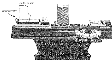
SK313型 200針 (パンチカード方式) KR3型 ニットレーダー
